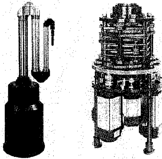
Figura 2.6. Telemanipulador TELBOT junto con la caja de transmisión por engranajes situada en su base. (Cortesía de Wälischmiller GmbH.)
