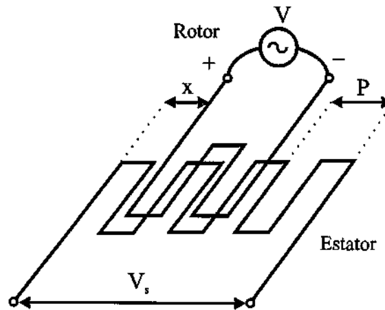
Figura 2.24. Esquema de funcionamiento de un Inductosyn.
