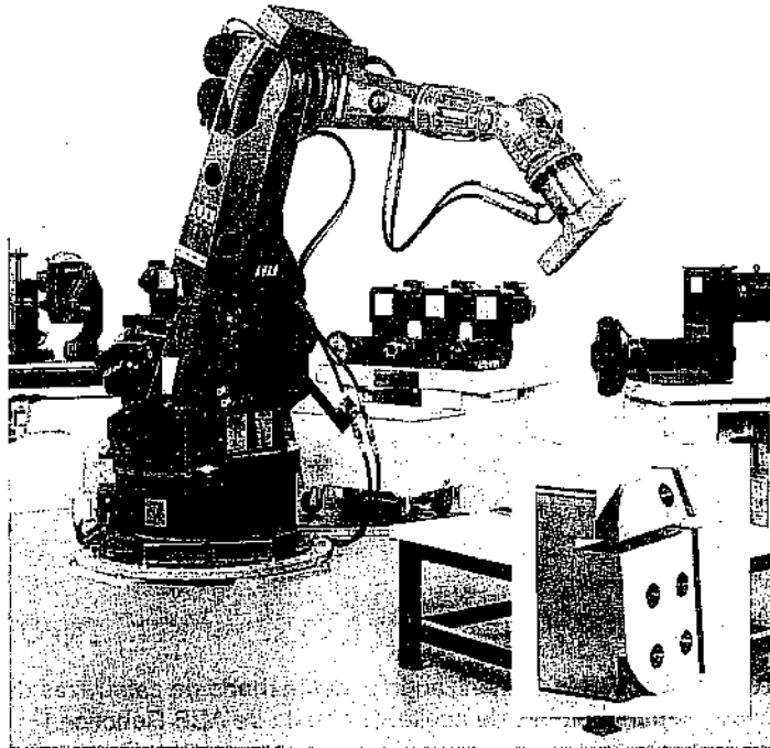
Figura 10.7. Robot IR 761/125.0 en célula de tratamiento (fresado, taladrado, serrado, etc.) de componentes de aluminio. (Cortesía de KUKA.)
