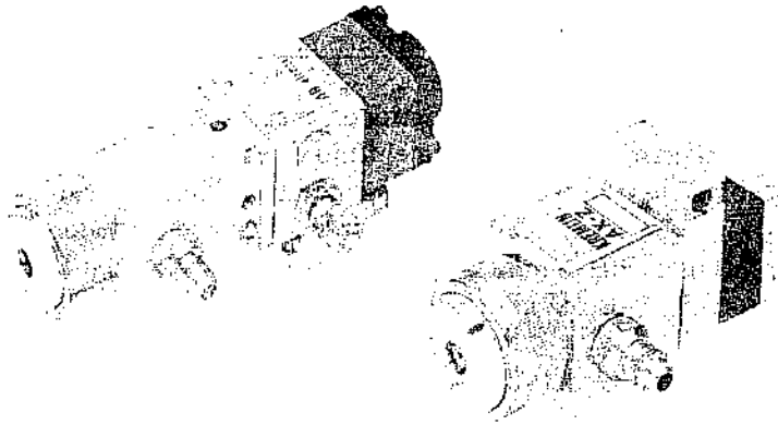
Figura 2.26. Pistolas neumáticas de pulverización de pintura. (Cortesía de Kremlin.)
