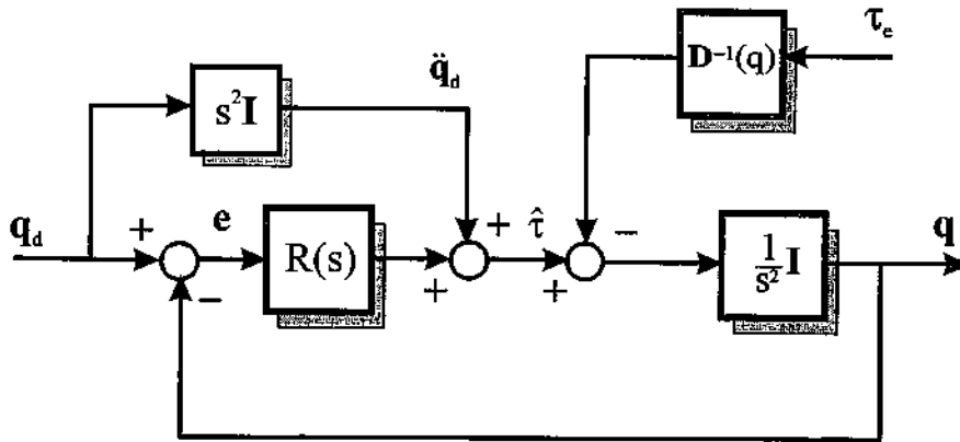
Figura 7.11. Esquema de algoritmo de control basado en PID y prealimentación sobre el sistema desacoplado.
