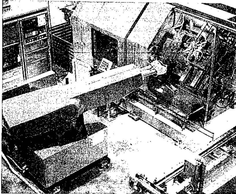
Figura 1.2. Robot Unimate 2000. Uno de los primeros modelos comerciales de Unimation. (Cortesía de Staübl.)
