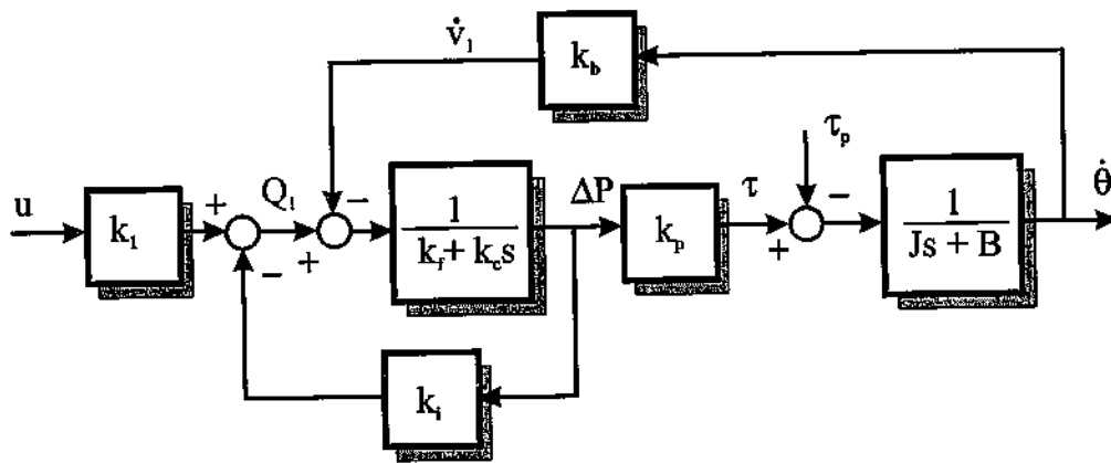
Figura 5.12. Diagrama de bloques del modelo de actuador hidráulico.
