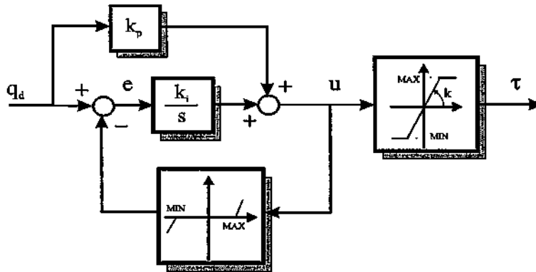
Figura 7.21. Control monoarticulado con regulador PID antiwind-up .
