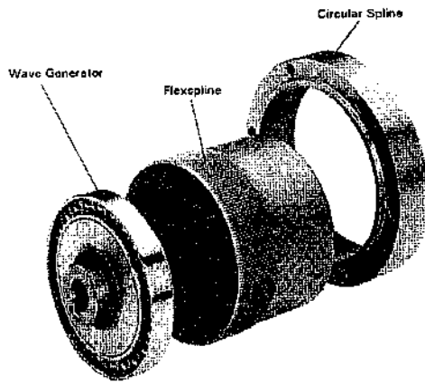
Figura 2.7. Despiece HDUC. (Cortesía de HarmonicDrive.)
